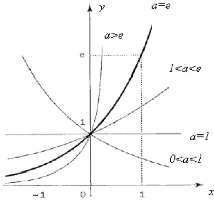
FIGURE 4. Graphe de la fonction y = a^x
