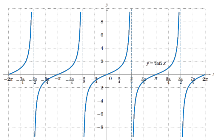
FIGURE 3. Graphe de la fonction \tan x
