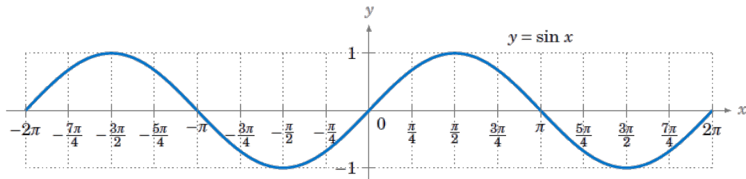
FIGURE 1. Graphe de la fonction \sin x
