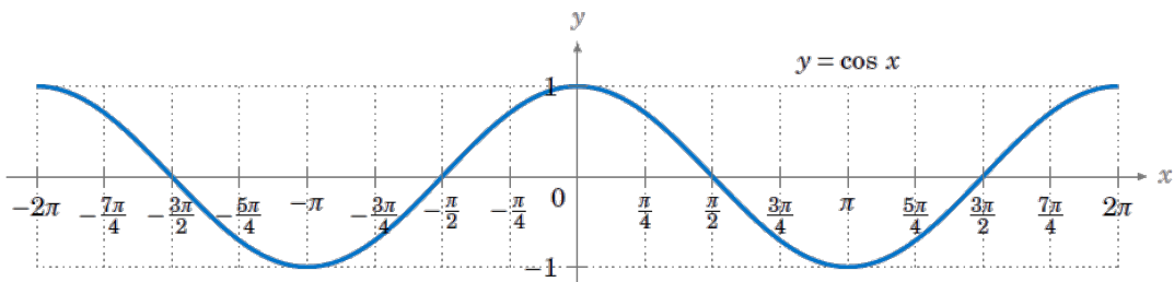
FIGURE 2. Graphe de la fonction \cos x
