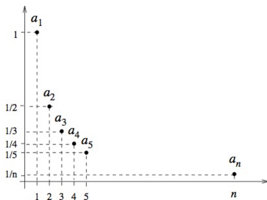
FIGURE 1. Représentation graphique de la suite \{1/n\}_{n=1}^\infty
