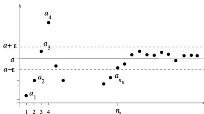
FIGURE 2. Suite convergent à a
